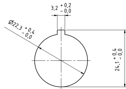
Einbaumaße/dimensions
